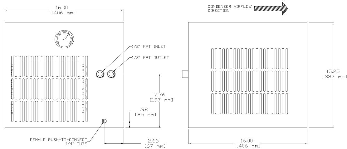
MODEL VF-15 DIMENSIONS
